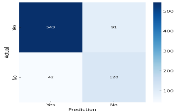
Gambar 4. Confusion Matrix untuk NB
