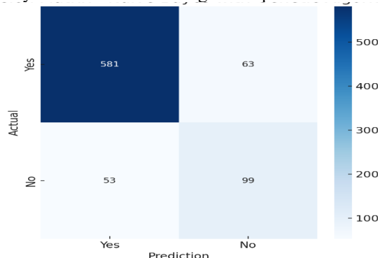
Gambar 6. Confusion Matrix untuk NB dengan GA
