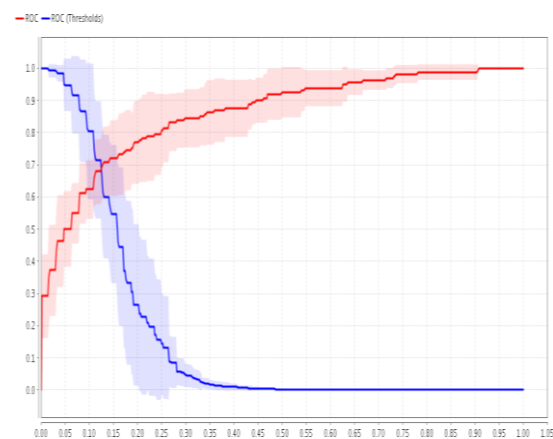
Gambar 5. AUC Model NB
